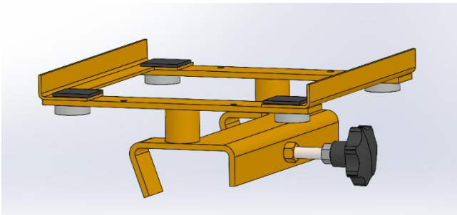
Sans entretoise : Hauteur position basse (70±5mm)
