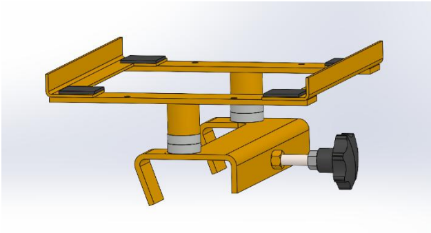
Avec 4 entretoises : Position haute (90±5mm)
